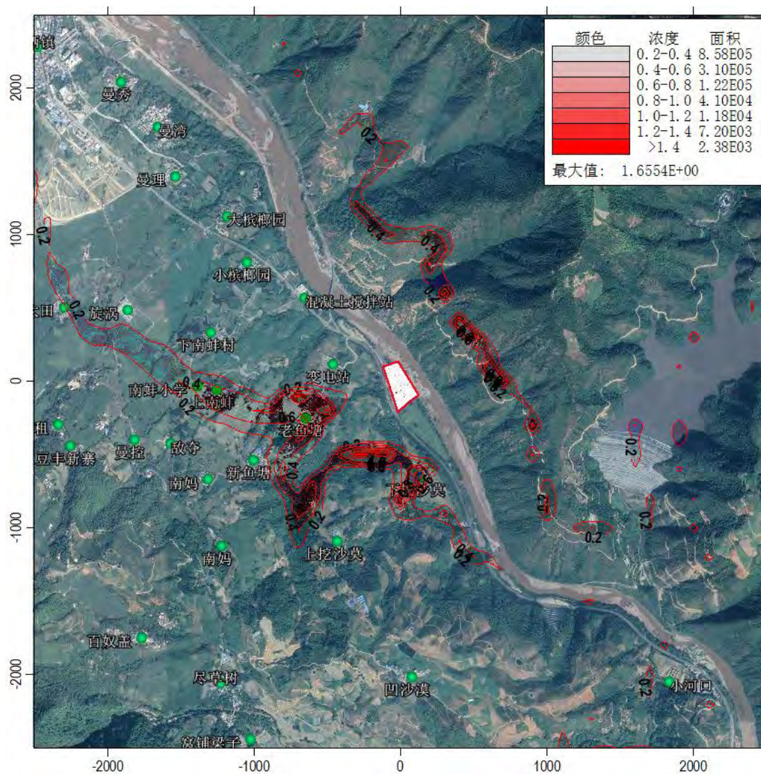
图 5.2.4-13 HCl 小时质量浓度贡献值分布图 ( \mu\text{g}/\text{m}^3 )
