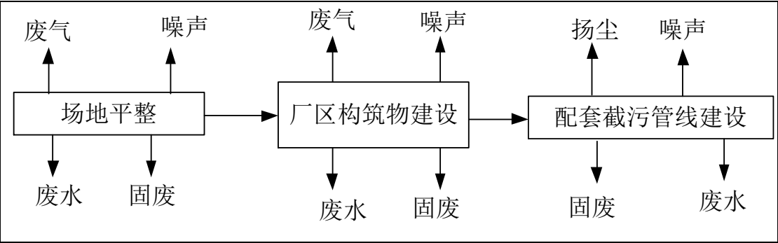
图 3.2-1 施工工艺及产污环节示意图
