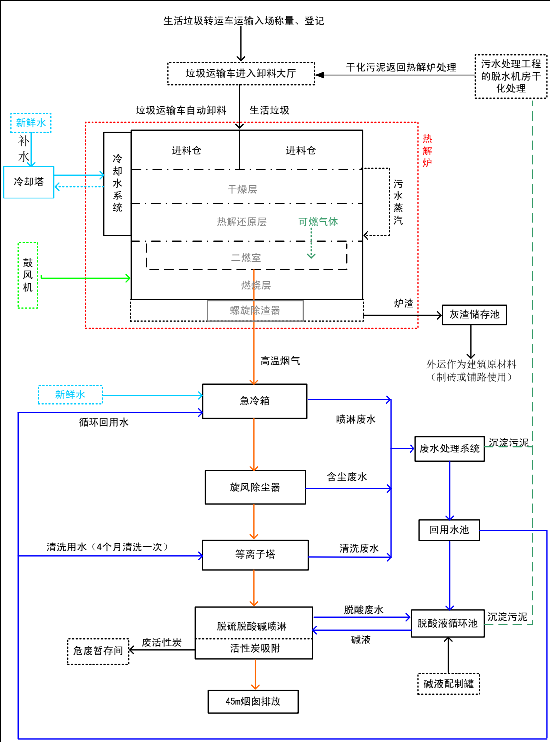
图 3.3-5 项目工艺流程及产污节点示意图
