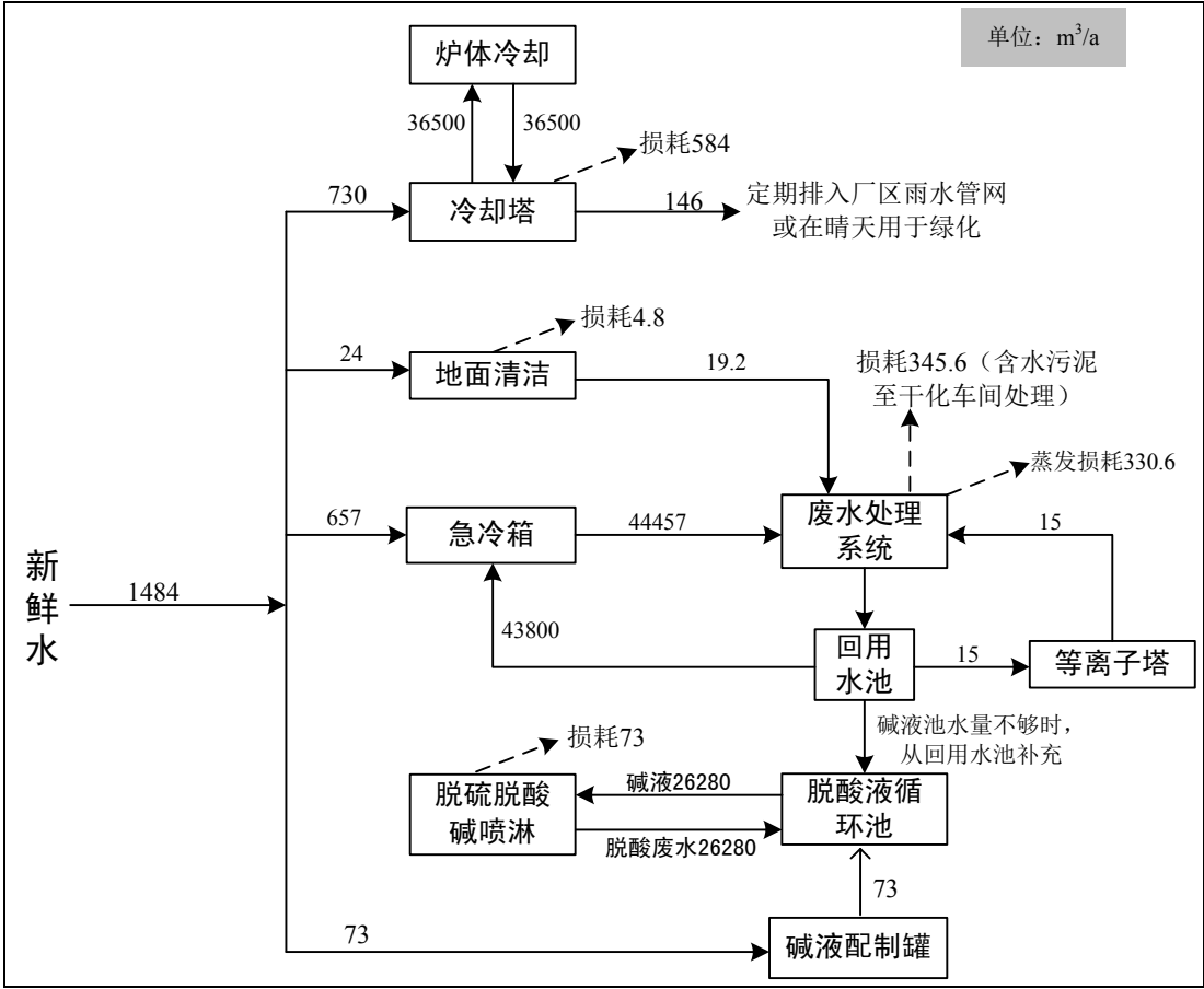
图 3.3-7 项目垃圾热解工程水平衡图
