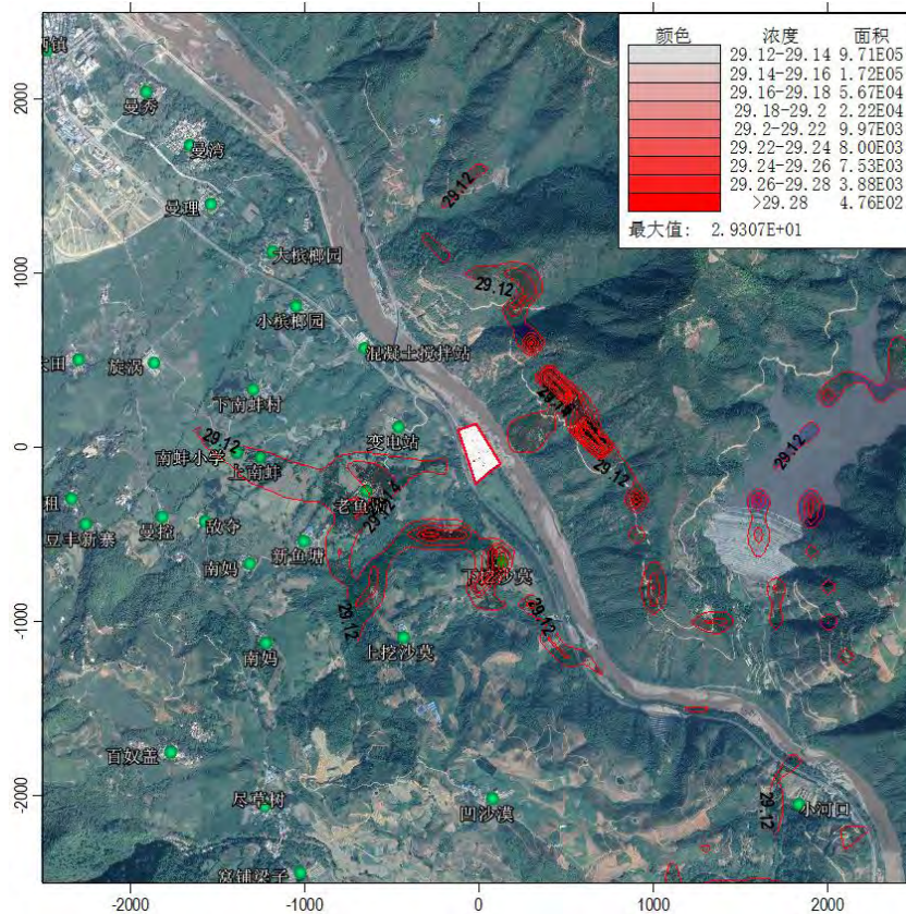
图 5.2.4-7 PM 10 95%保证率日均质量浓度分布图 (μg/m 3 )
