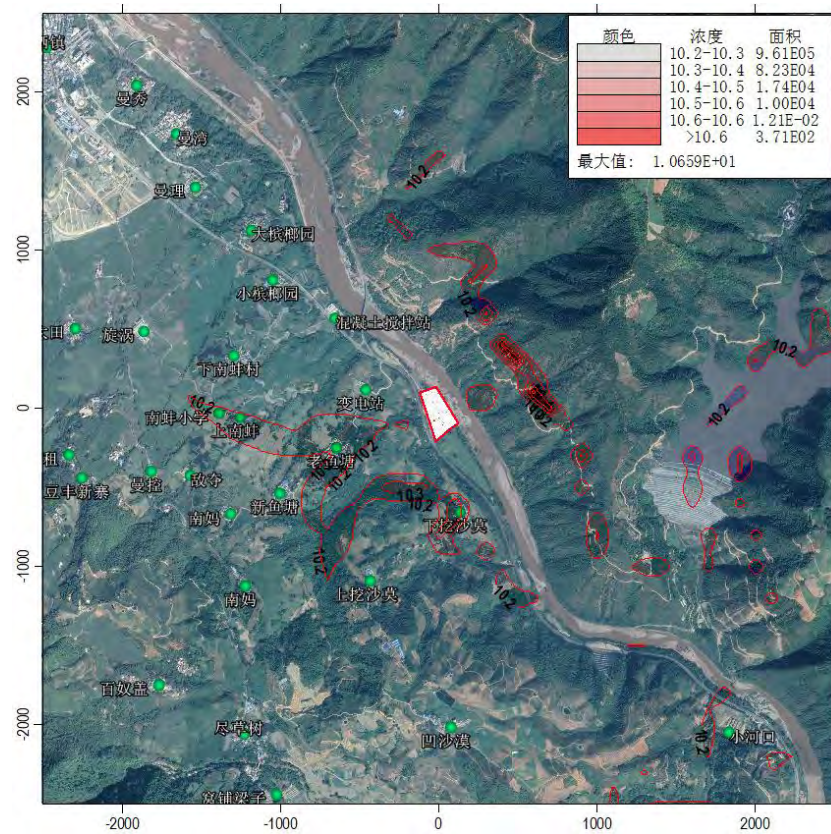
图 5.2.4-1 \text{NO}_2 98%保证率日均质量浓度分布图 ( \mu\text{g}/\text{m}^3 )
