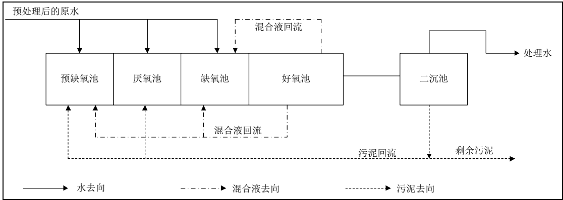
图 3.3-9 本项目 A 2 /O 工艺流程示意图
