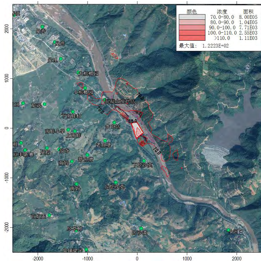
图 5.2.4-15 NH 3 小时质量浓度分布图 (μg/m 3 )
