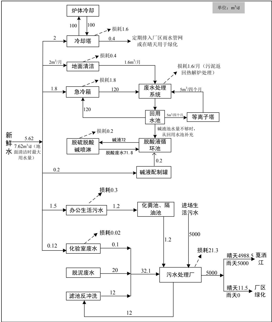
图 3.4-1 项目总水量平衡图
