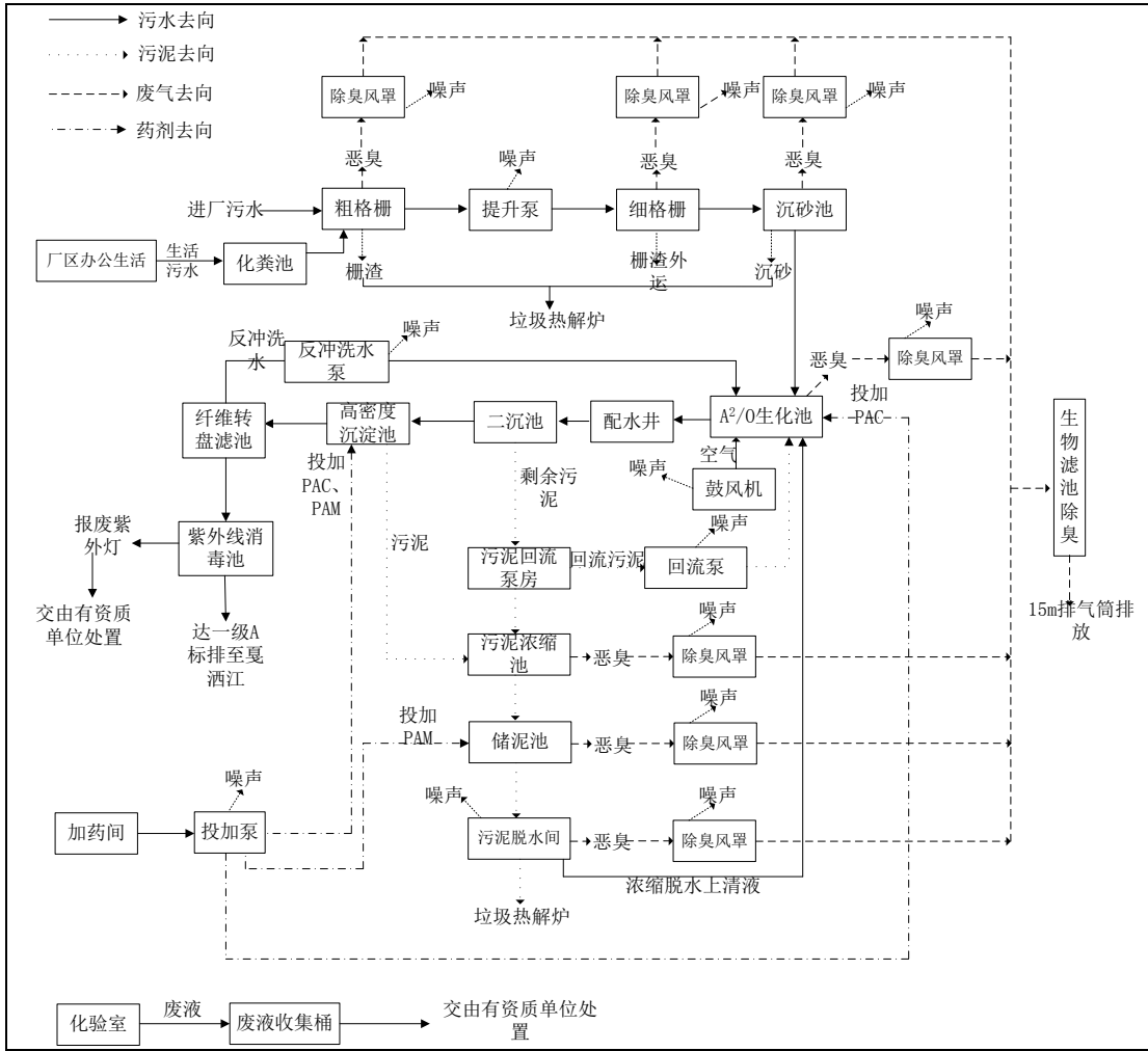
图 3.3-8 新平戛洒镇污水处理厂工艺流程及产污节点图
