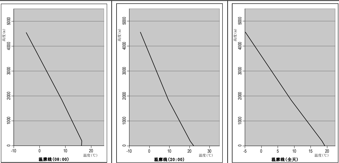
图 5.2.2-6 温廓线
