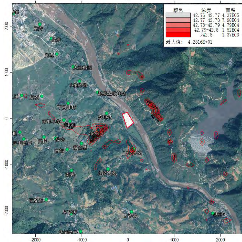
图 5.2.4-9 PM 2.5 95%保证率日均质量浓度分布图 (μg/m 3 )
