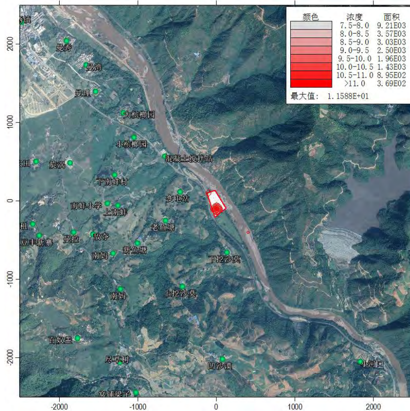
图 5.2.4-16 H_2S 小时质量浓度分布图 ( \mu g/m^3 )
